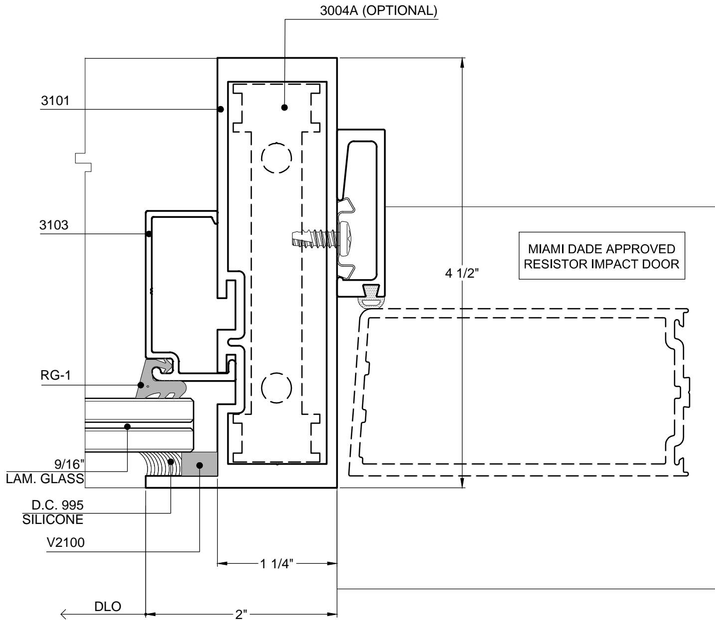
40A DOOR JAMB
